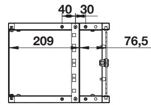
KESİT C-C
