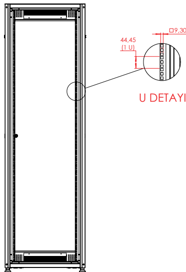
GENİŞLİK VE YÜKSEKLİK ÖLÇÜLERİ
