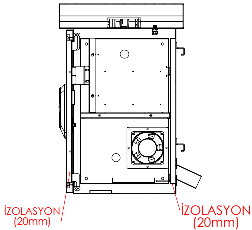
YAN KESİT GÖRÜNÜŞ
