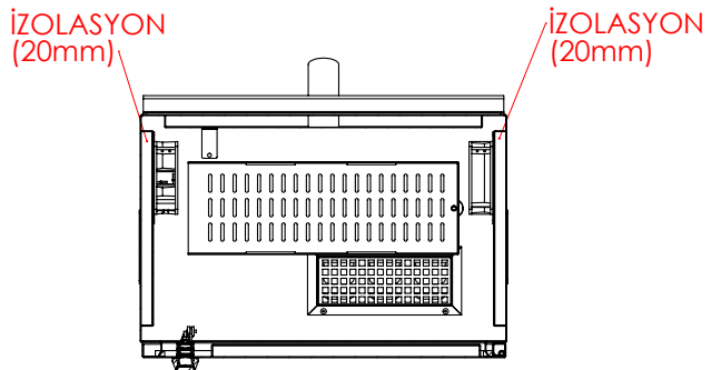
ÜST KESİT GÖRÜNÜŞ
